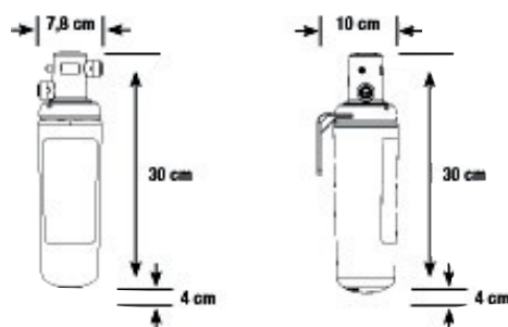
rozměry 3M filtrační patrony
